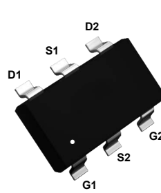
SOT-23-6L
